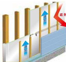
【外断熱工法】
