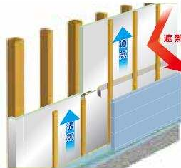
【外断熱工法】
